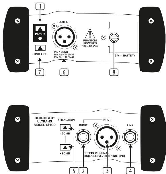
DI100 の前部および後部
