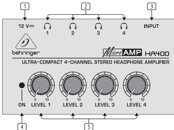
Betjeningselementer og tilslutninger på HA400
