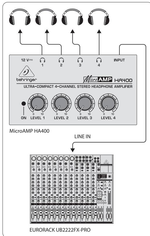
Ledningsføring for HA400
