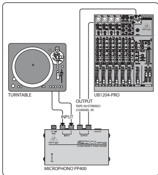
PP400 の結線
