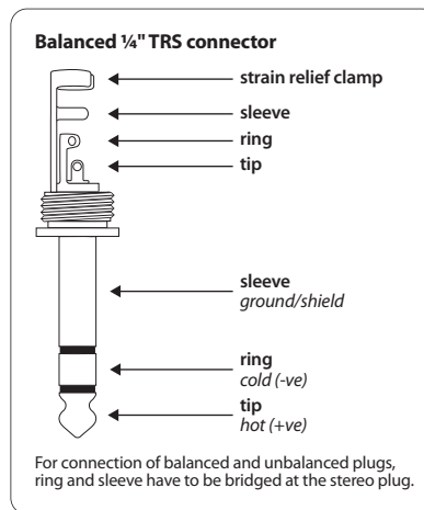
Fig. 4.1: Jack stéréo 6,3 mm
