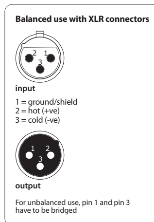
Fig. 4.2: Liaisons XLR
