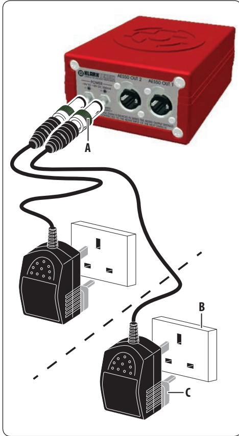
Typischer zweifach redundanter Netzanschluss. A. Verriegelbarer Netzteil-Anschluss. B. Netzsteckdose (britische Version). C. Landesspezifischer Steckeradapter (britische Version).
