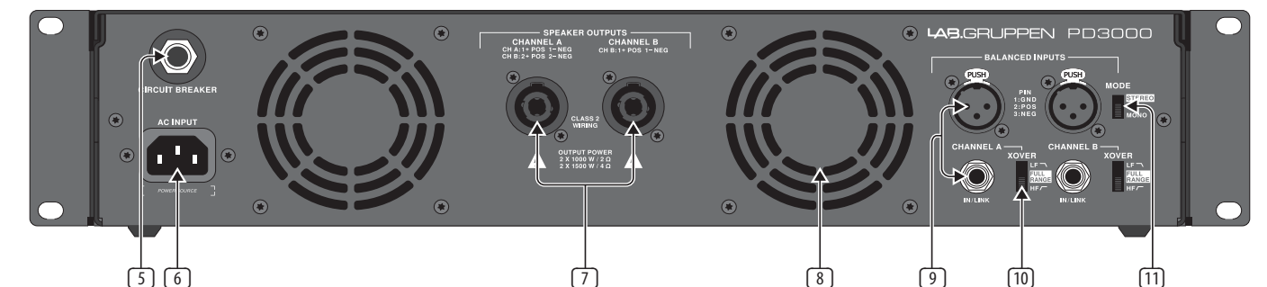
Afb. 2: PD3000 Achterpaneel
