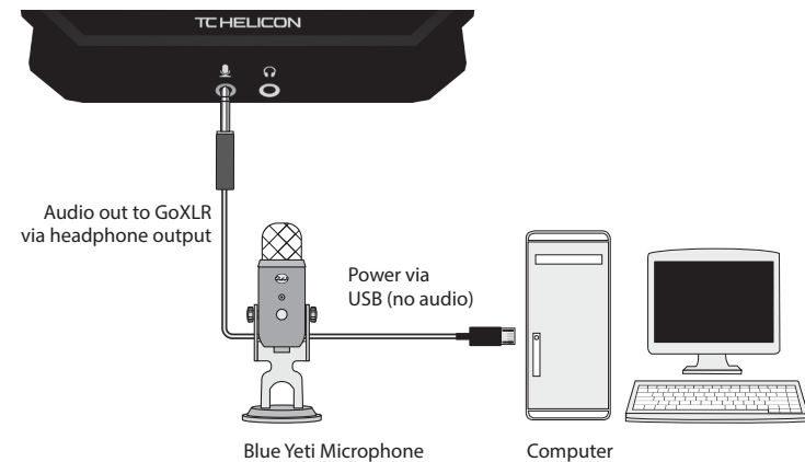
Connexion recommandée du Blue Yeti Mic
