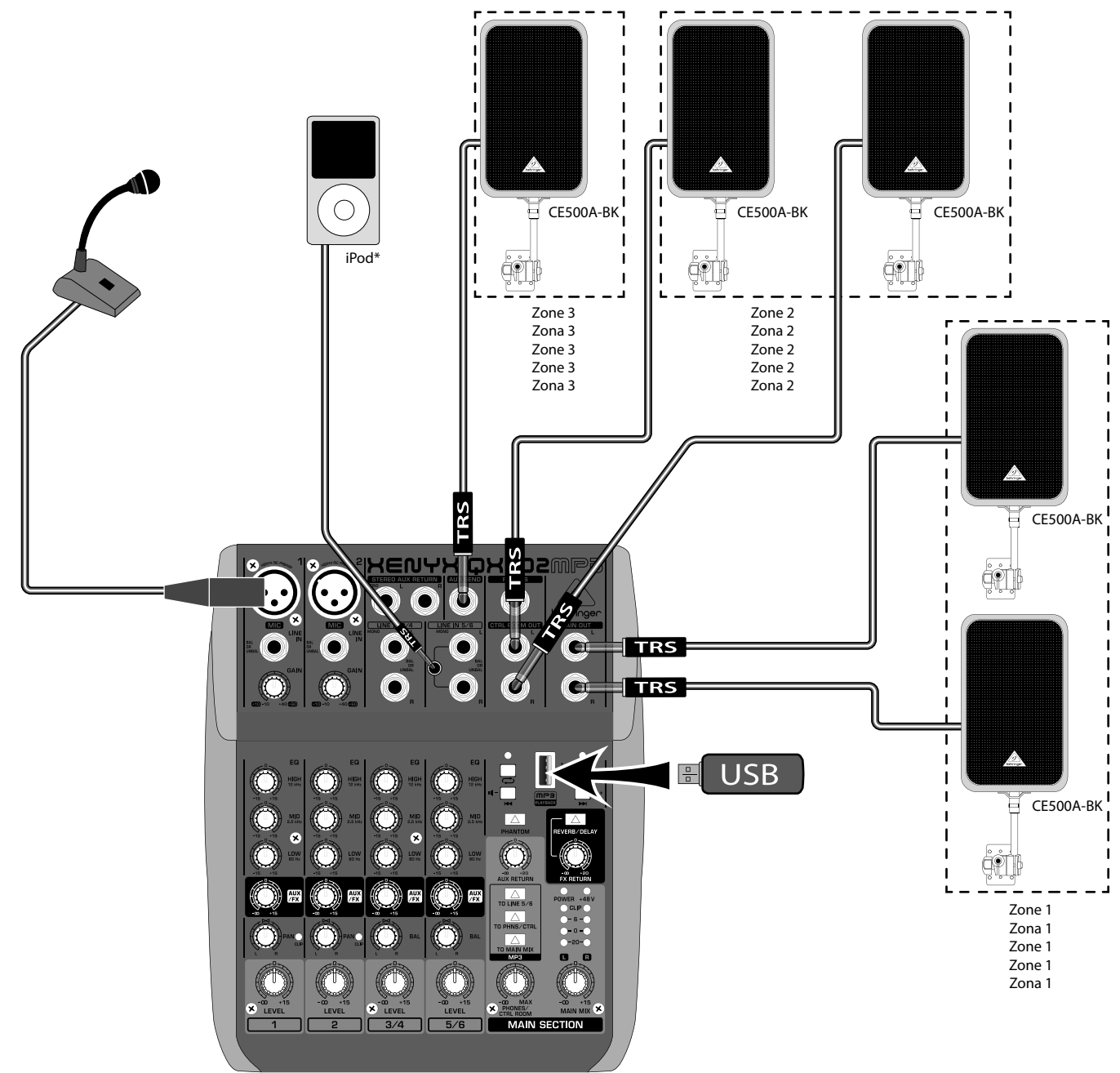
Small shop/restaurant sound system with MP3 playback, additional iPod audio, microphone and speakers set up in 3 independent zones. Sistema de sonido para pequeño comercio/restaurante con reproducción MP3, audio iPod adicional, micrófono y altavoces configurado en 3 zonas independientes. Sonorisation d'un petit magasin/restaurant avec diffusion de MP3, audio en provenance d'un iPod, micro et enceintes placées dans 3 zones différentes. Für kleine Läden/Restaurants geeignetes Soundsystem mit MP3-Wiedergabe, zusätzlichem iPod-Audio, Mikrofon und in 3 unabhängigen Zonen aufgestellten Lautsprechern Sistema de som para pequenas lojas/restaurantes com playback de MP3, áudio iPod adicional, configuração de microfone e alto-falantes em 3 zonas independentes.
