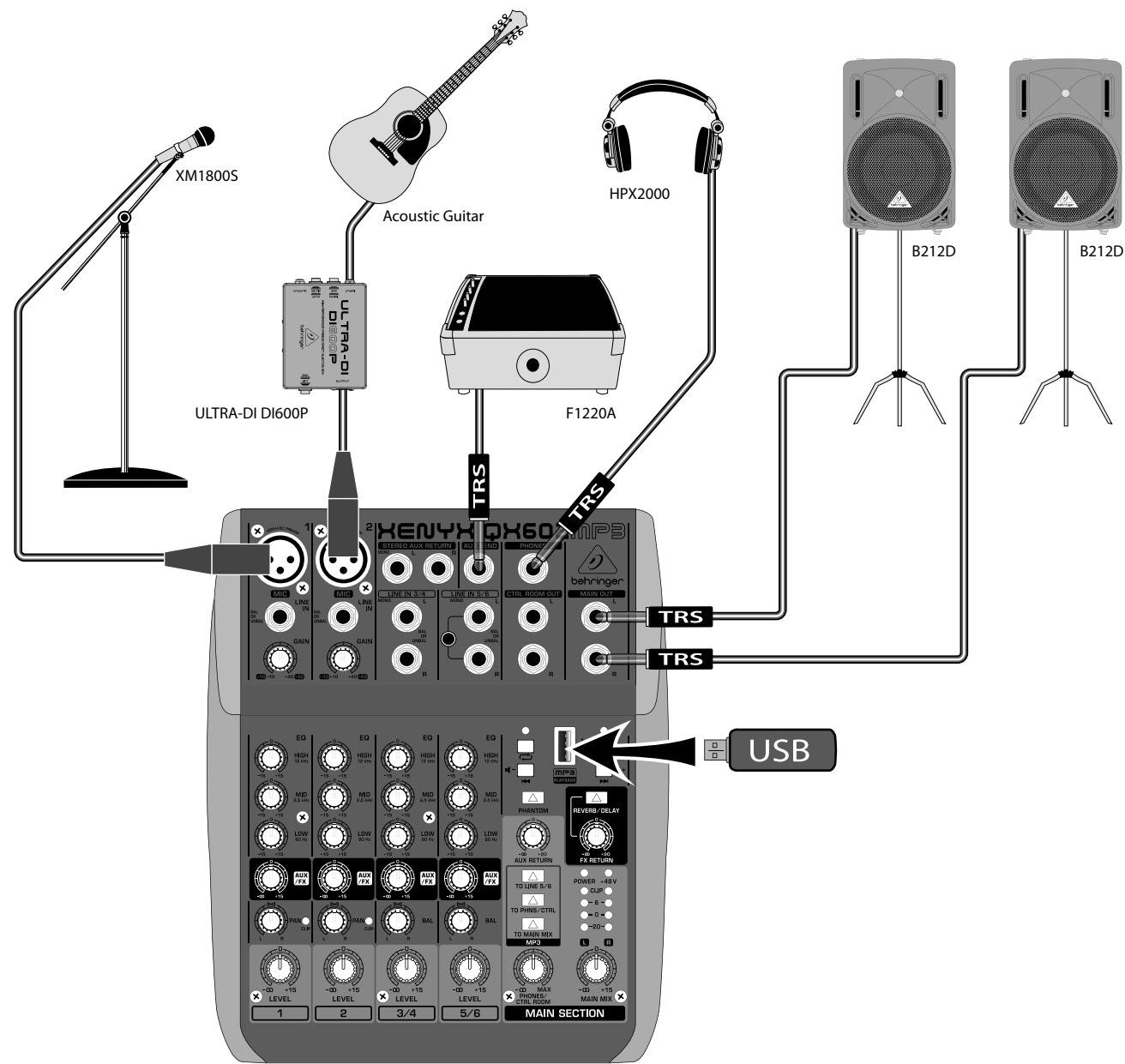
Singer-songwriter setup with MP3 backing tracks Configuración para compositor-cantautor con pistas de acompañamiento en MP3 Configuration pour chanteur-compositeur avec accompagnement en MP3 Singer-Songwriter Setup mit MP3-Begleitspuren Configuração para cantor-compositor com faixas de fundo MP3
