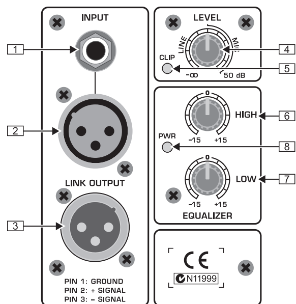
Fig. 2.1: Commandes et connexions (B212A et B215A)
