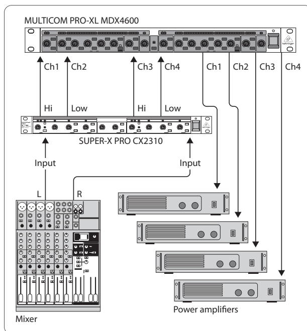
図 4.3: MDX4600 によるマルチバンド・コンプレッション
