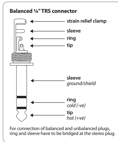
図 5.3: 6.3 mm ステレオフォンプラグ
