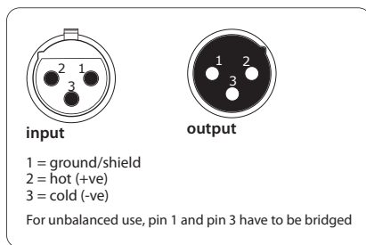
図 5.1: XLR 接続
