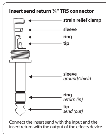
図 5.4: インサートケーブル用 6.3 mm ステレオフォンプラグ
