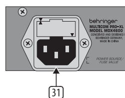
図 2.7: 電圧供給およびヒューズ
