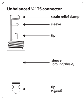
図 5.2: 6.3 mm モノラルフォンプラグ
