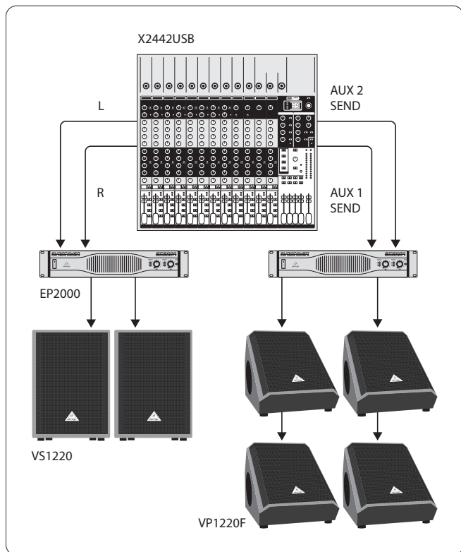
Εικ. 5.2: Στερεοφωνική λειτουργία με επιδαπέδια μόνιτορ
