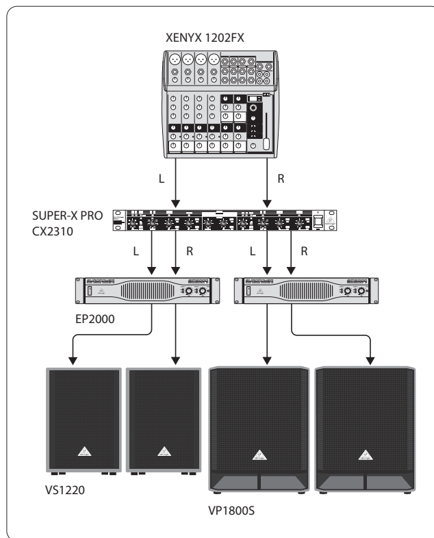
Εικ. 5.3: Αμφίδρομη στερεοφωνική λειτουργία με subwoofer
