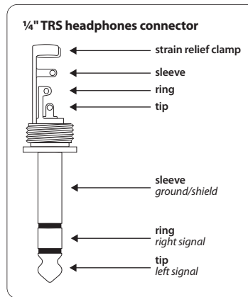
图 3.4: 耳机立体声插头
