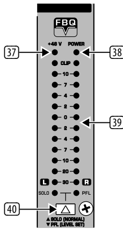
Εικ. 2.16: Ποτενσιόμετρο Main Out
