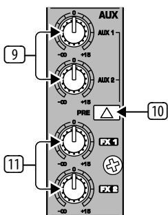
Εικ. 2.3: Ρυθμιστές AUX/FX Send στους διαύλους
