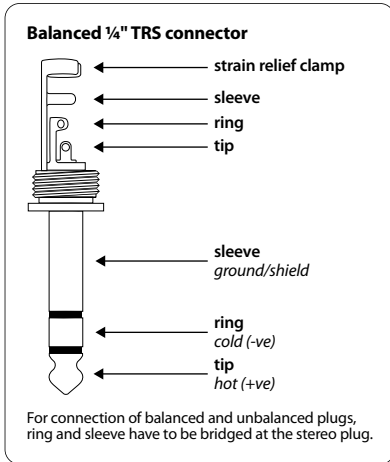
Εικ. 5.2: Στερεοφωνικό βύσμα 6,3 mm
