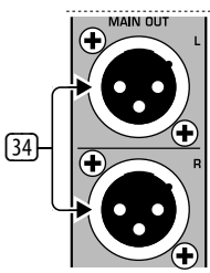
Εικ. 2.14: Έξοδοι XLR-Main Out
