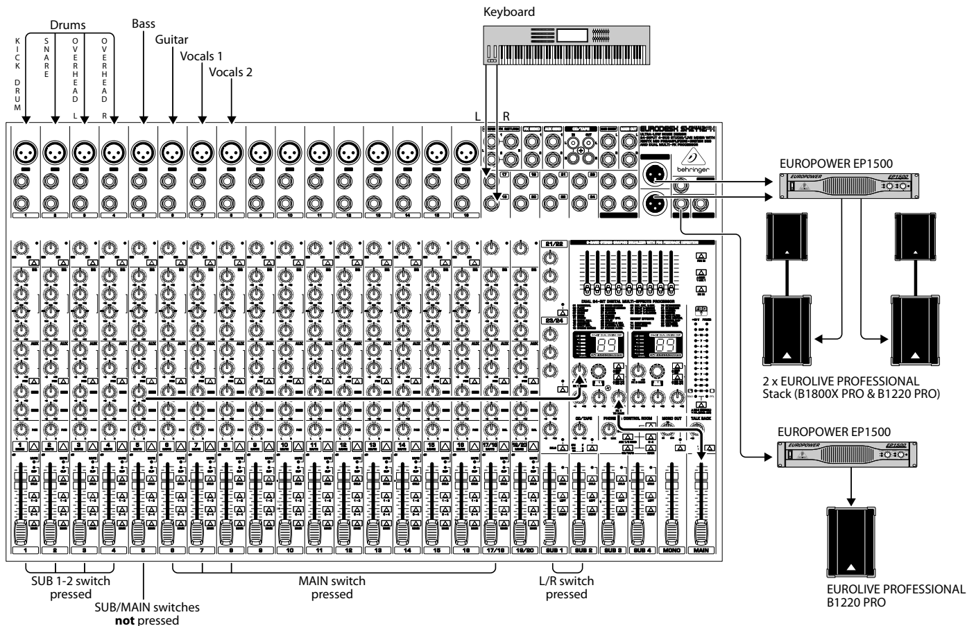
Εικ. 4.2: Καλωδίωση κονσόλας μείξης στη λειτουργία Live
