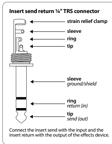
Εικ. 5.7: Στερεοφωνικό βύσμα Insert-Send-Return
