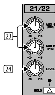
Εικ. 2.8: Πρόσθετα στερεοφωνικά κανάλια
