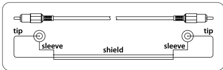
Εικ. 5.3: Καλώδιο Cinch
