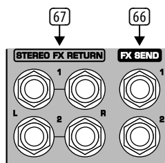
Εικ. 2.26: Συνδέσεις FX Send και Return
