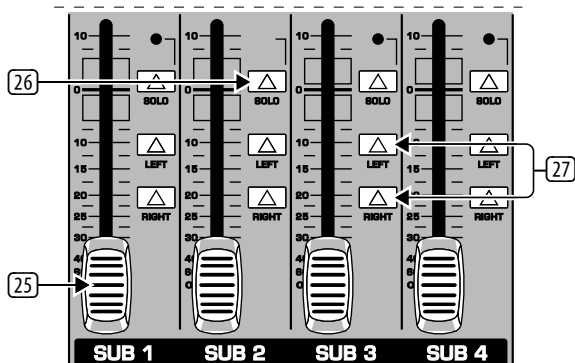
Εικ. 2.9: Οι υποομάδες 1-4
