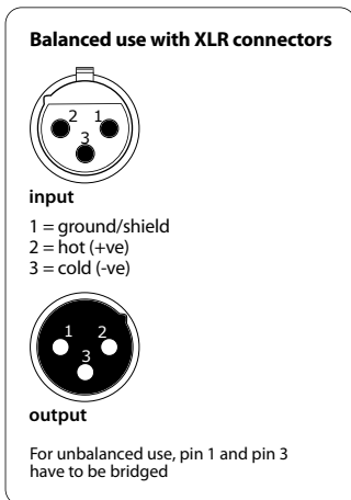
Εικ. 5.4: Συνδέσεις XLR
