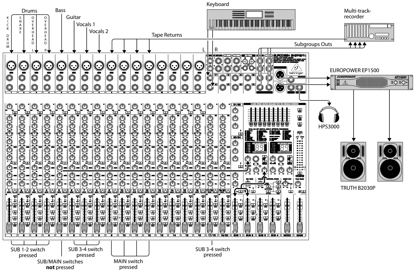
Εικ. 4.1: Καλωδίωση κονσόλας μείξης κατά τη λειτουργία Studio
