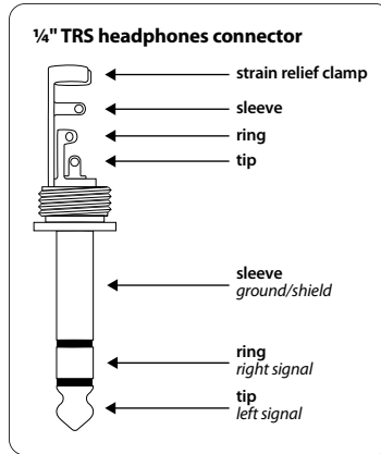
Εικ. 5.6: Στερεοφωνικό βύσμα ακουστικών
