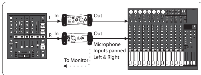
Abb. 2.2: DJ-Mixer \Rightarrow 2 x DI-Box \Rightarrow Mischpult
