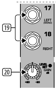
Afb. 2.5: De stereo-kanaalingangen
