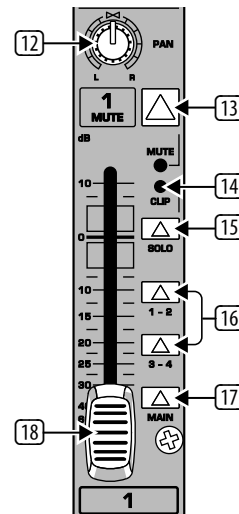
Afb. 2.4: Kanaal-Fader, Pan-regelaar, Mute-schakelaar etc.
