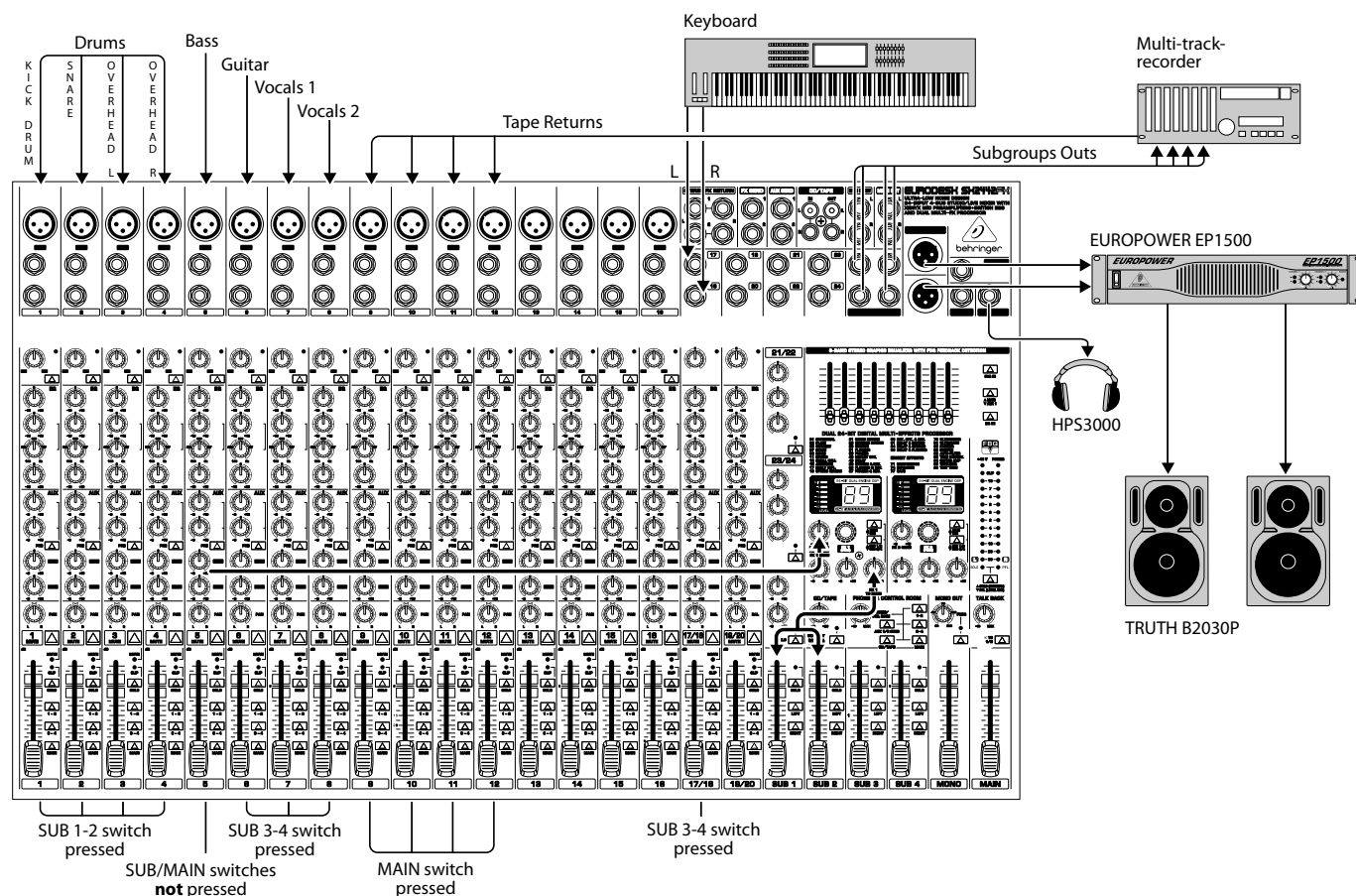
Afb. 4.1: Mengpaneelaansluitingen in Studio-opstelling
