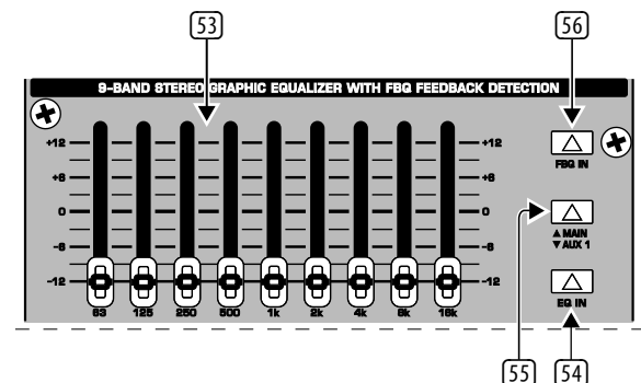
Afb. 2.24: De grafische stereo-equalizer
