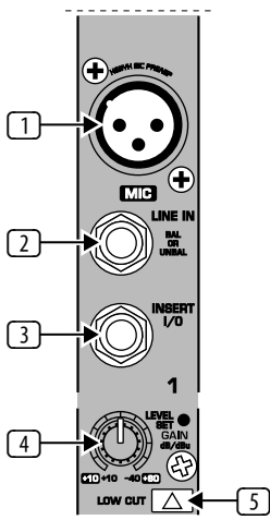
Afb. 2.1: Aansluitingen en regelaars van de Mic-/Line-ingangen
