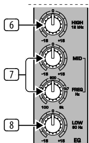
Afb. 2.2: De klankregeling van de ingangskanalen
