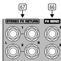
Afb. 2.26: FX Send- und Return-aansluitingen
