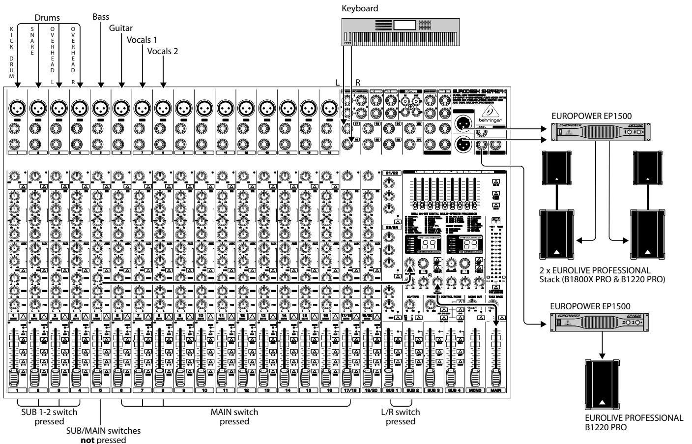
Afb. 4.2: Mengpaneelaansluitingen in Live-opstelling
