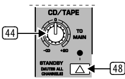
Afb. 2.20: CD/Tape
