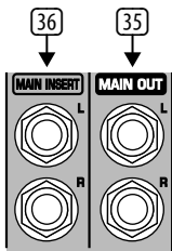
Afb. 2.15: Main Out-Klinkeruitgangen en Main Insert
