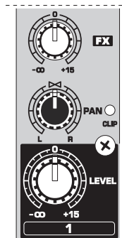
図. 2.3: FX センド / パノラマ / レベルコントローラー
