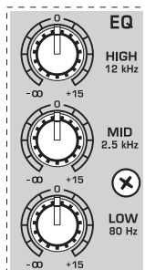
図. 2.2: モノラル入力チャンネルのサウンドコントロール
