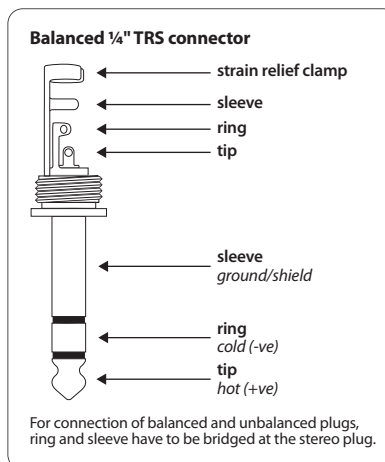
図. 3.3: 6.3 mm ステレオフォンプラグ
