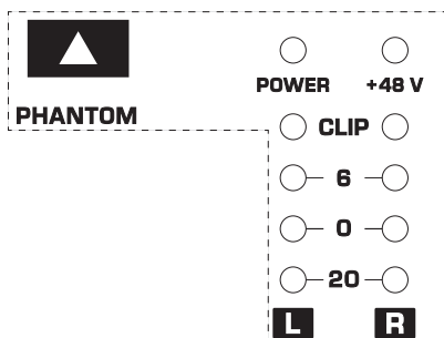
図. 2.13: ファントム電源供給および各コントロール LED
