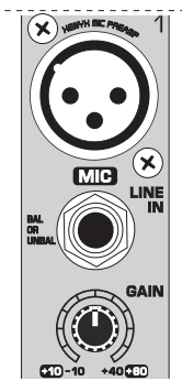
図. 2.1: マイク入力およびライン入力の各接続端子とコントローラー
